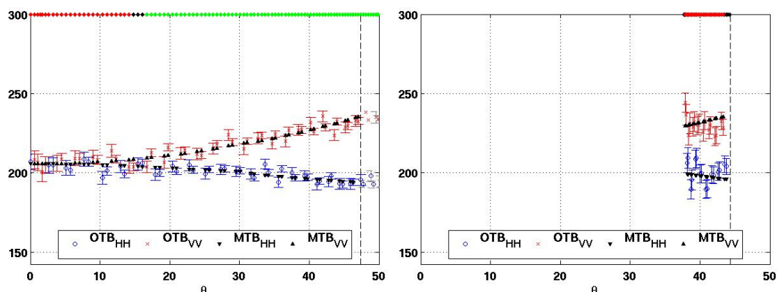
Figure 1 : profil de températures de brillance [K] (couleur) observées par SMOS, modélisation inverse (noir) en fonction de la géométrie (angle d'incidence \theta ) et variabilité d'échantillonnage angulaire et magnitude du bruit (barre d'erreur) pour le même point observé mais sous différente géométrie, sous-trace du satellite (gauche), bord de champ de vue (droite)
