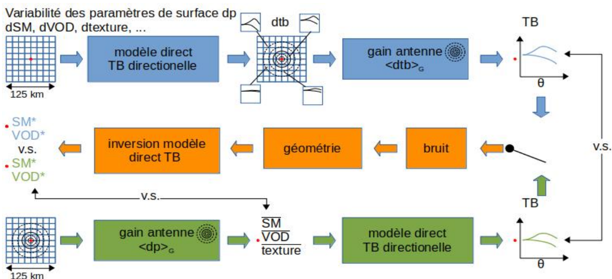
Figure 2 : aperçu conceptuel de l'exercice de modélisation : schémas directs (ici deux types bleu, vert) : paramètres géophysiques ( dSM , dVOD , dtexture ) vers températures de brillance TB injectées dans un schéma inverse : températures de brillances, perturbées (bruit ajouté, signature angulaire, ...) vers paramètres géophysiques ( SM^* , VOD^* ).
